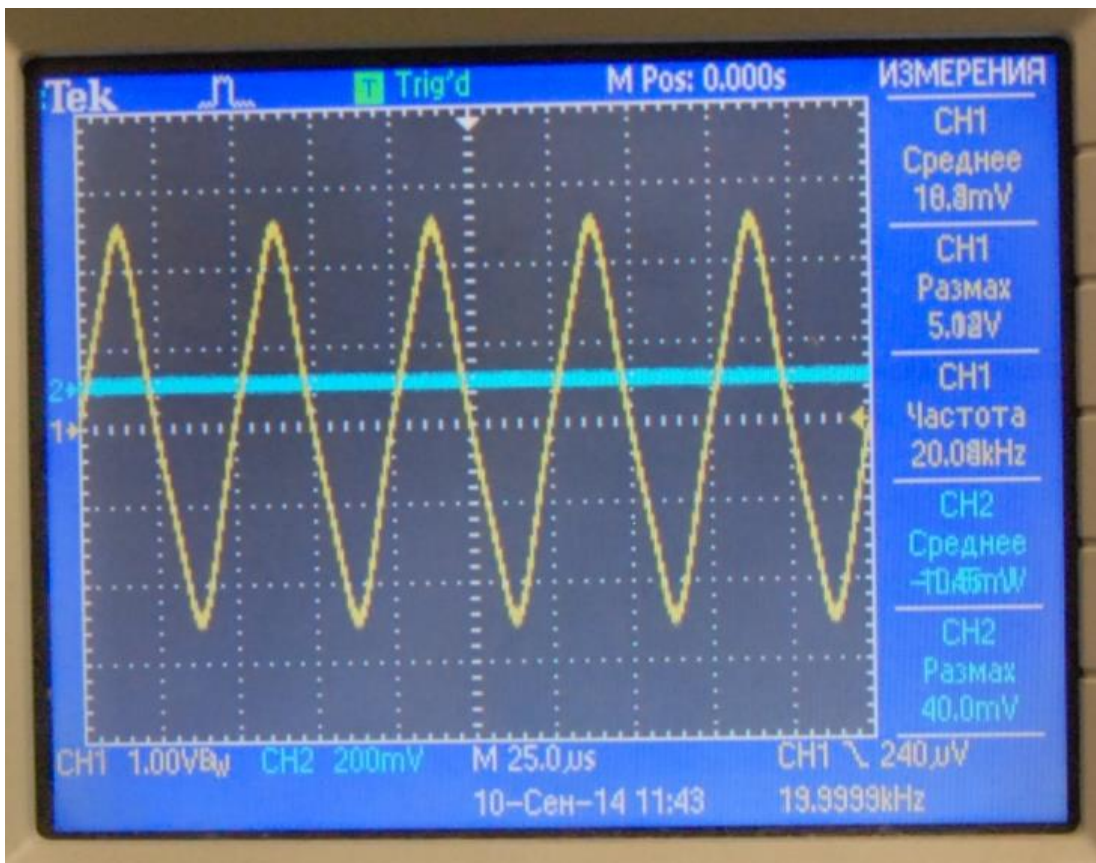
Треугольник 1кГц
