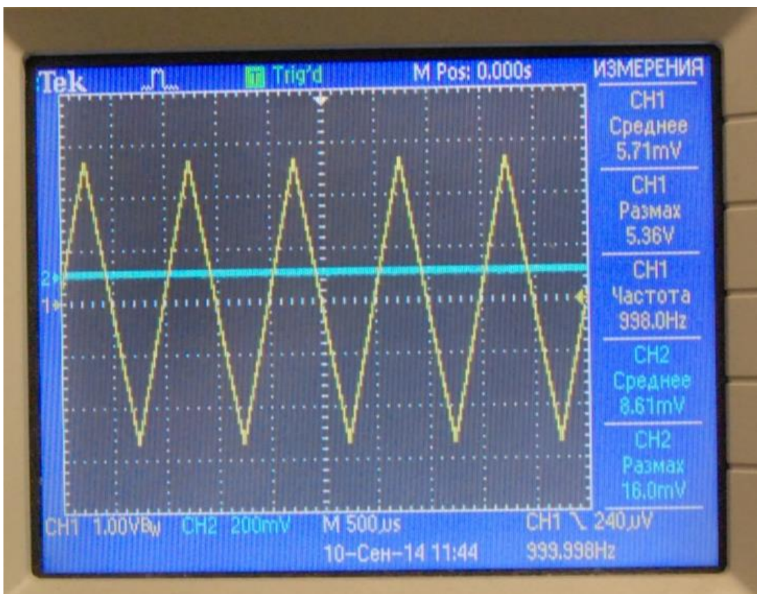
Гармоники на осциллографе. 1кГц первая (левый курсор). И правый курсор-третья. Разница 54дБ
