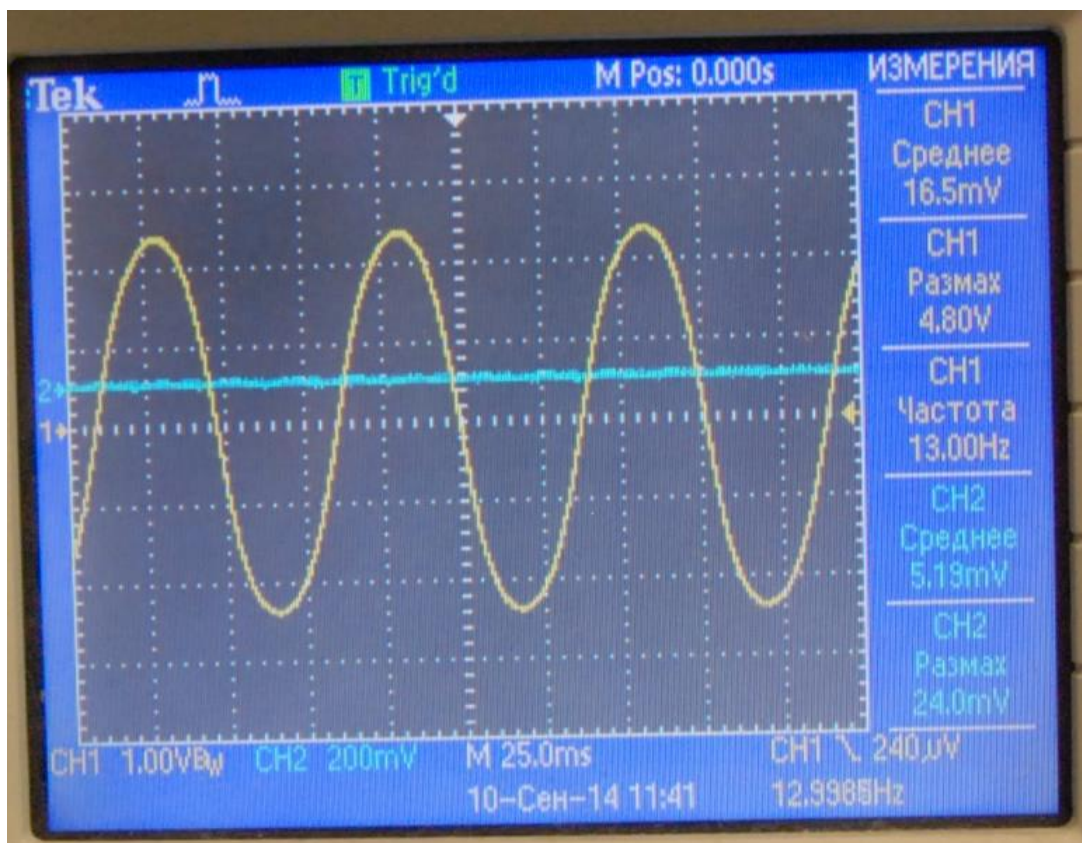
Синус 20кГц.
