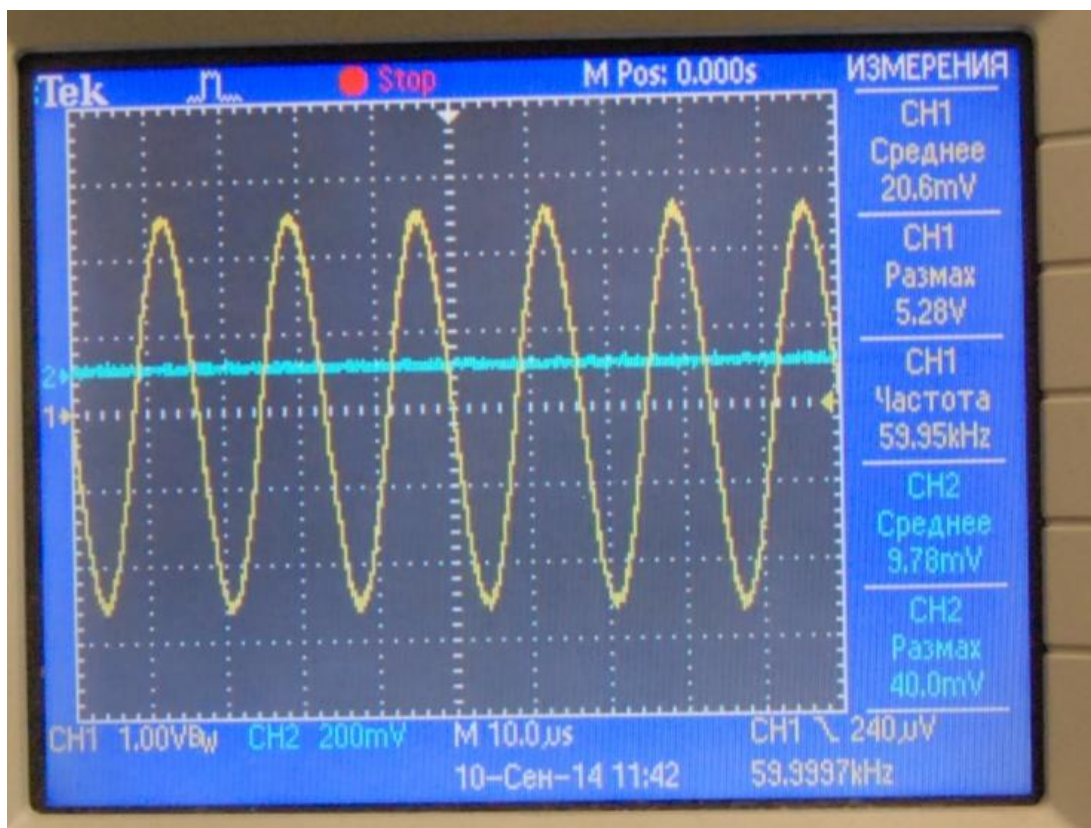
Синус 60кГц
