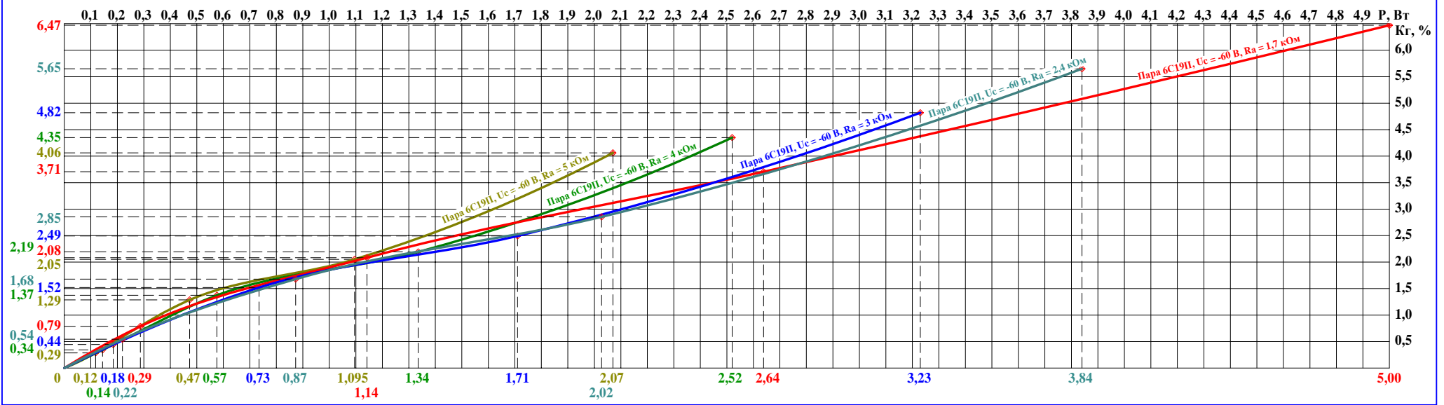
Зависимость искажений от выходной мощности для выходных каскадов на паре ламп 6С19П (при U_c = -60 В и R_a = 1700, 2426, 3000, 4000, 5000 Ом)
