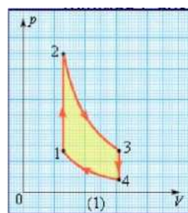
карбюраторный двигатель
