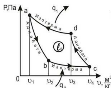
Обратный цикл Карно
