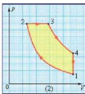
дизельный двигатель
